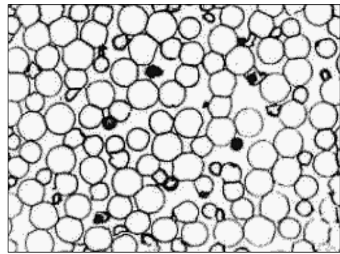
Polysphäre, teilverschäumt
